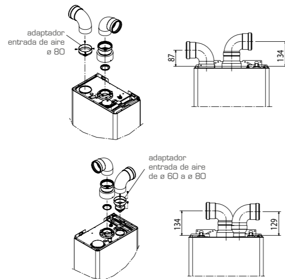
CONDUCTOS SEPARADOS PARA SALIDA HUMOS / ASPIRACIÓN AIRE Ø 80
